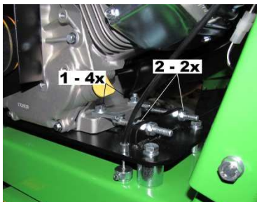
Fixation du moteur sur le châssis, F 360
