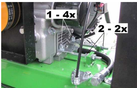
Fixation du moteur sur le châssis, F 460
