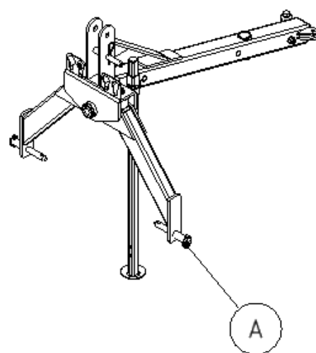
Závěs Kat. 1N Čelní
