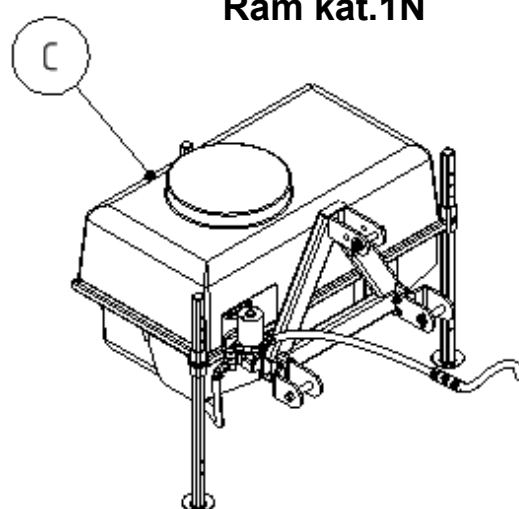
Rám TTR 4400
