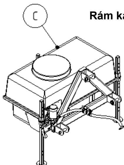
Rám TTR 4400
